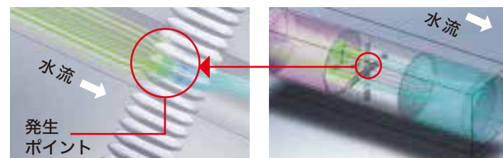
ハイスピードスピリエア (高速回転断部) さらに泡を超微細気泡にします。 キャビテーションポイント (発生装置部) ここでナノバブルを発生させます。
